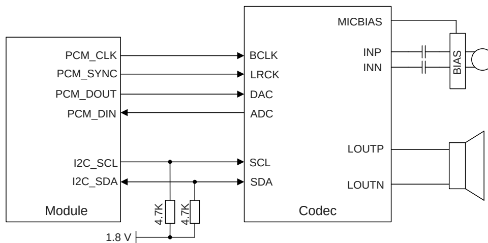
图 25: PCM 和 I2C 接口电路参考设计框图
