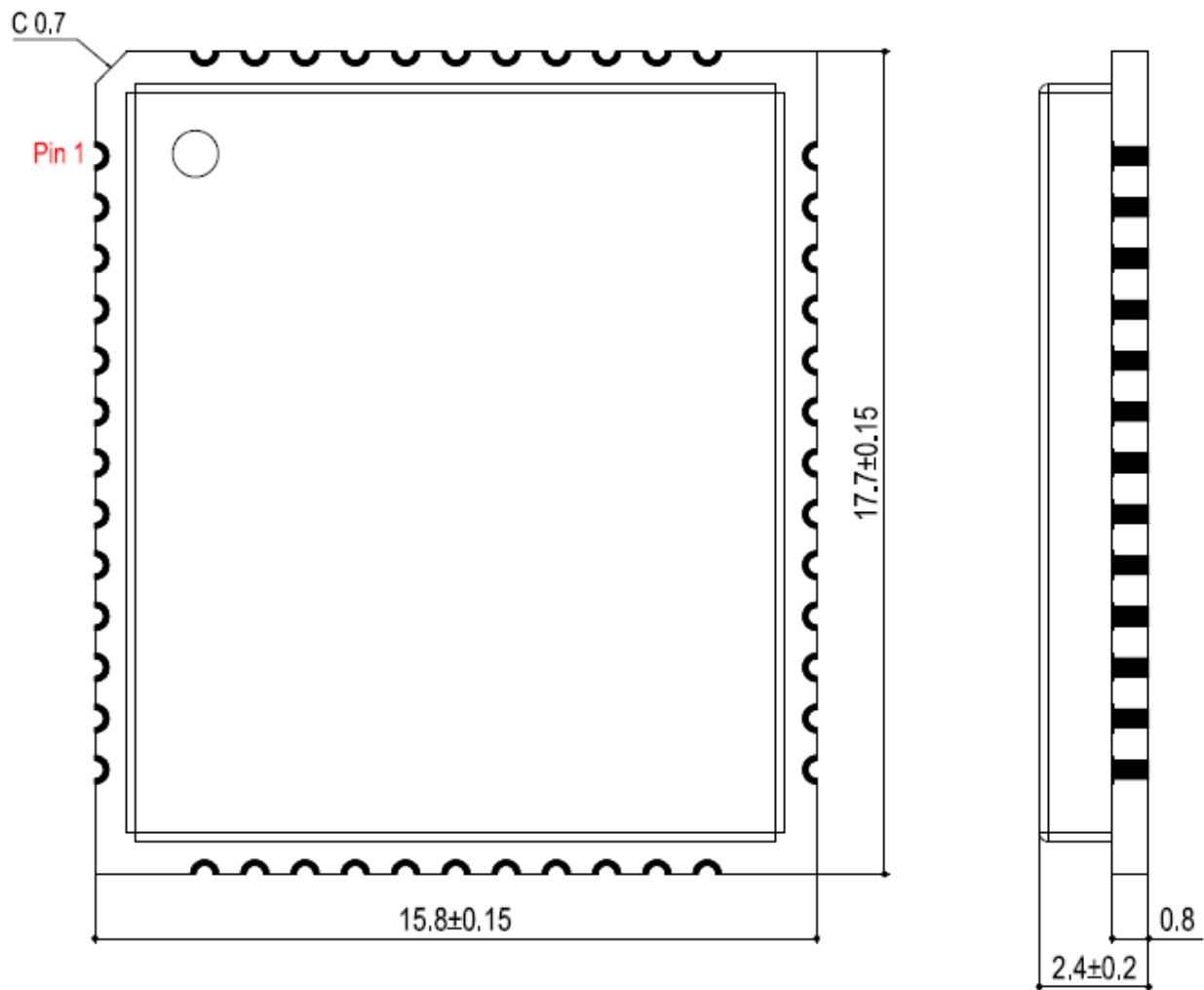
图 36：俯视及侧视尺寸图
