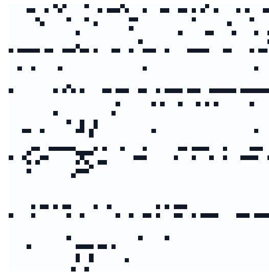
CCVM [MC]
