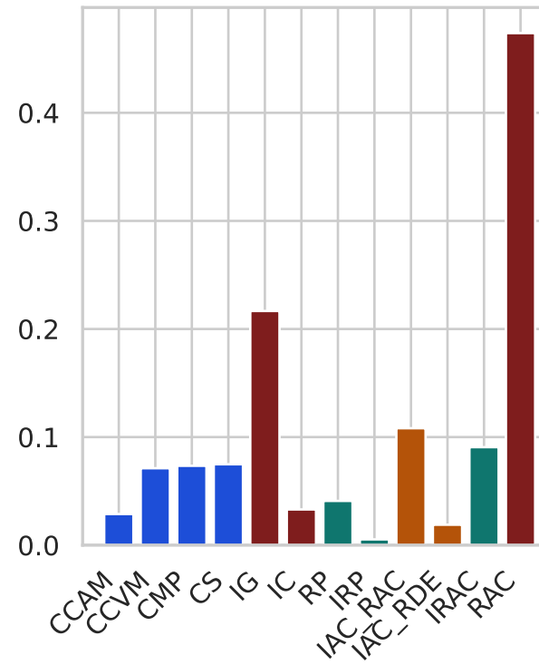
Edge density
