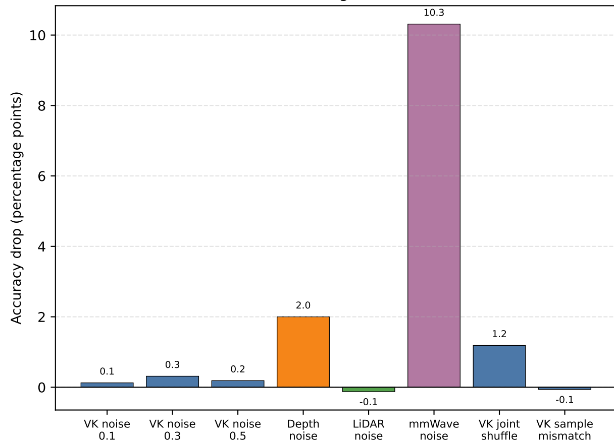
HAR diagnostic
