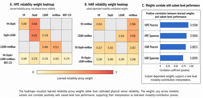
图 3: 模态子集上的学习可靠性代理权重。该权重是任务级贡献指标，不是校准的传感器健康度量。
