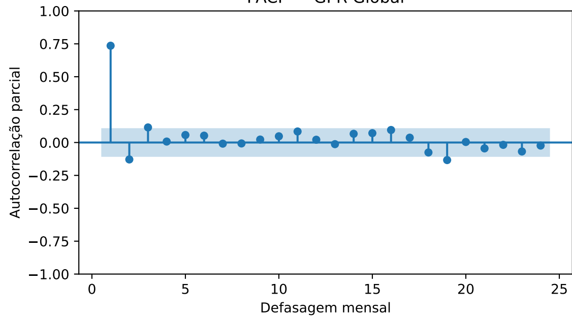
PACF — Log do GPR Global
