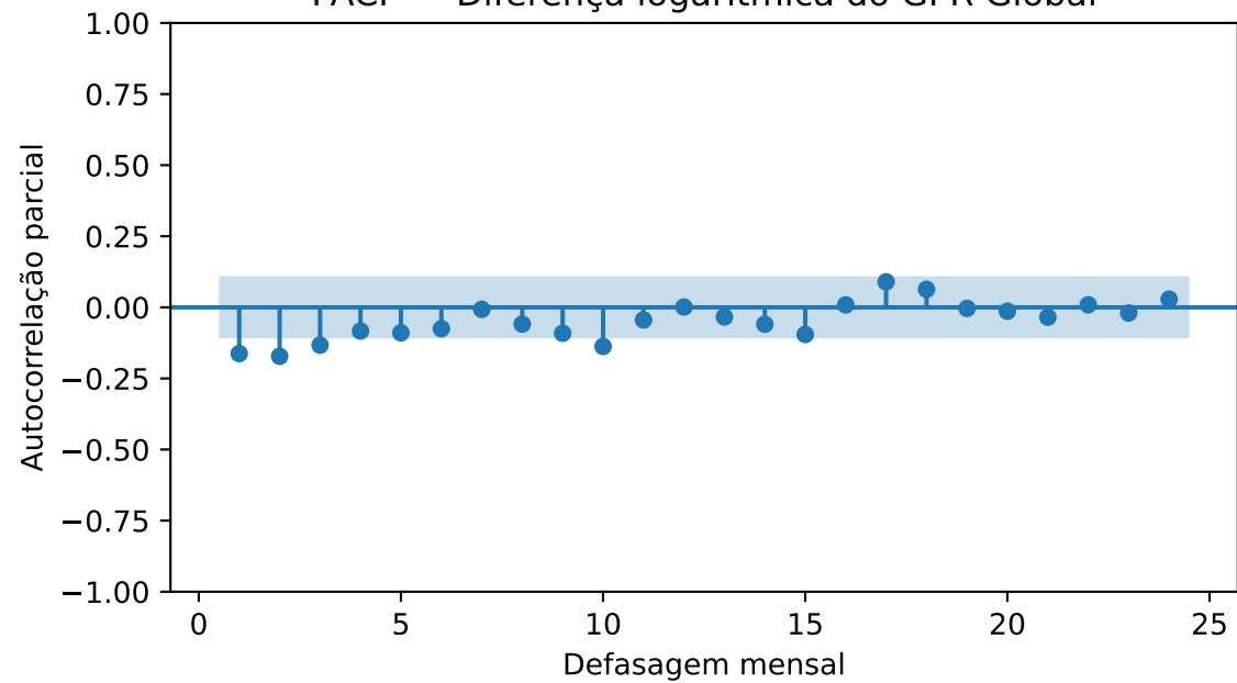
PACF — Diferença logarítmica do GPR Global
