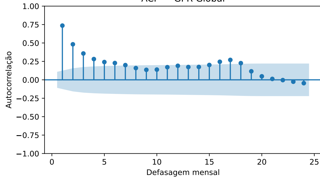
ACF — Log do GPR Global
