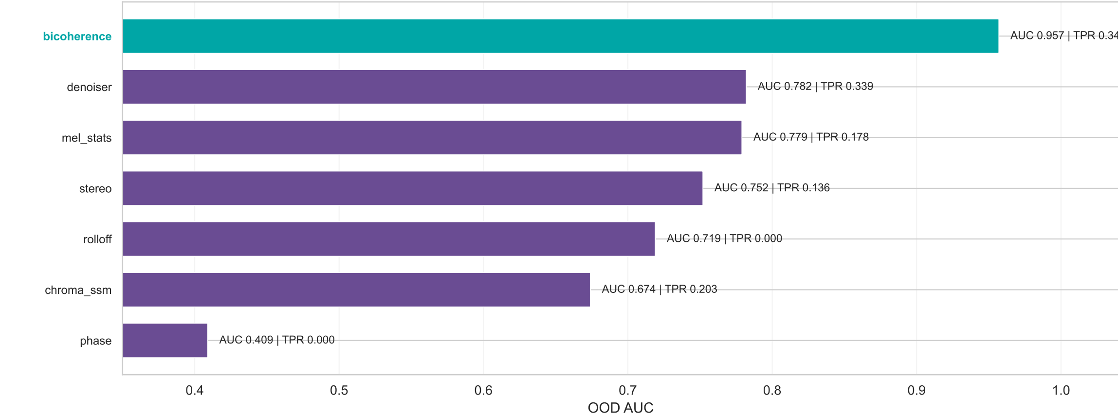
B. Standalone invariant probes
