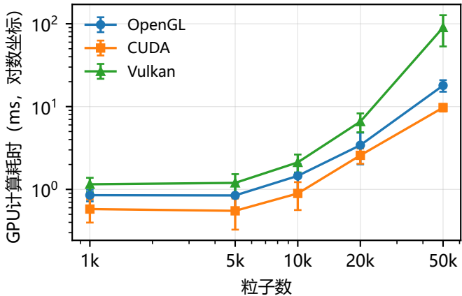
WCSPH
