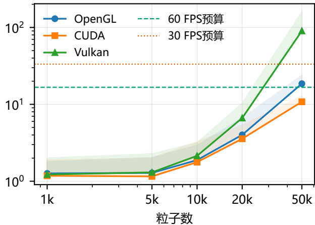
WCSPH
