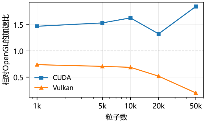
WCSPH
