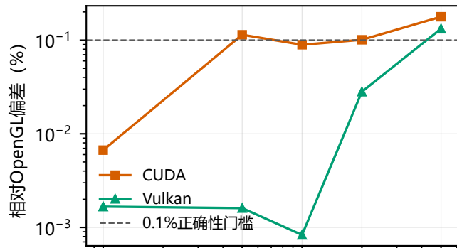
WCSPH: 相对偏差
