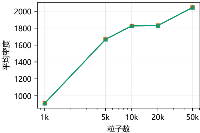
PCISPH: 平均密度
