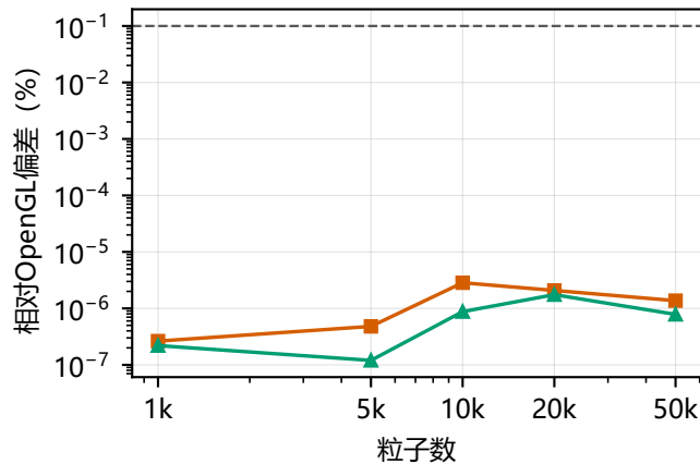
PCISPH: 相对偏差
