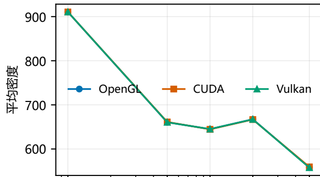
WCSPH: 平均密度
