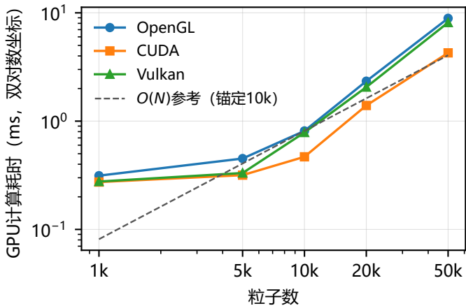
WCSPH
