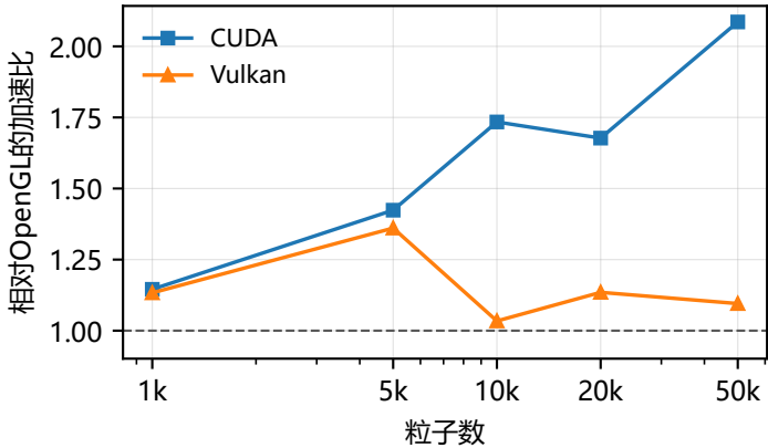
WCSPH
