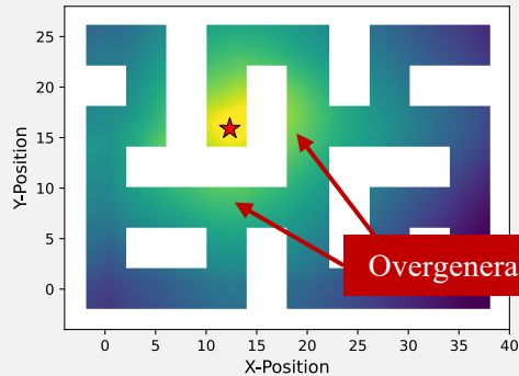
GCIVL + MLP
