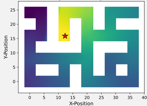
QRL + IQE
