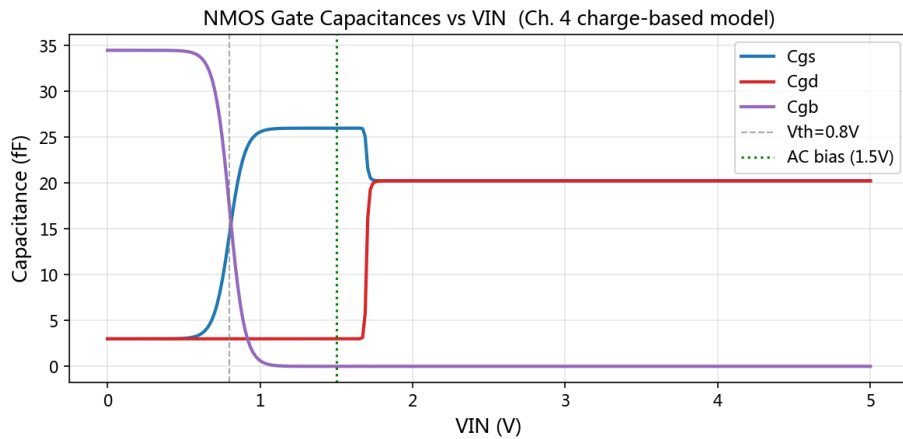
图 8: C_{gs} 、 C_{gd} 、 C_{gb} 随 VIN 的变化（含覆盖电容）
