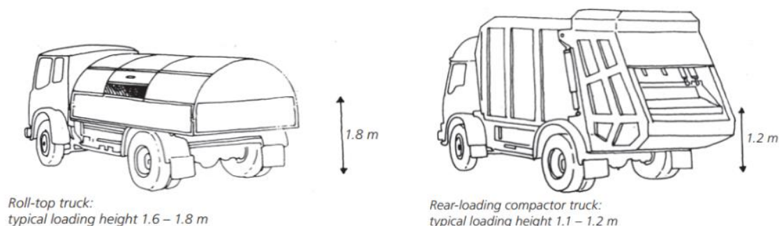
Figura 20 – Altura de carregamento dos veículos coletores de resíduos sólidos.
