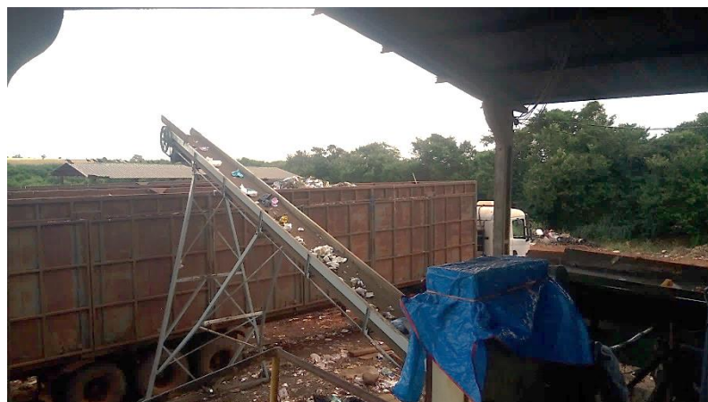
Figura 11 - Transbordo dos rejeitos em Caarapó-MS.
