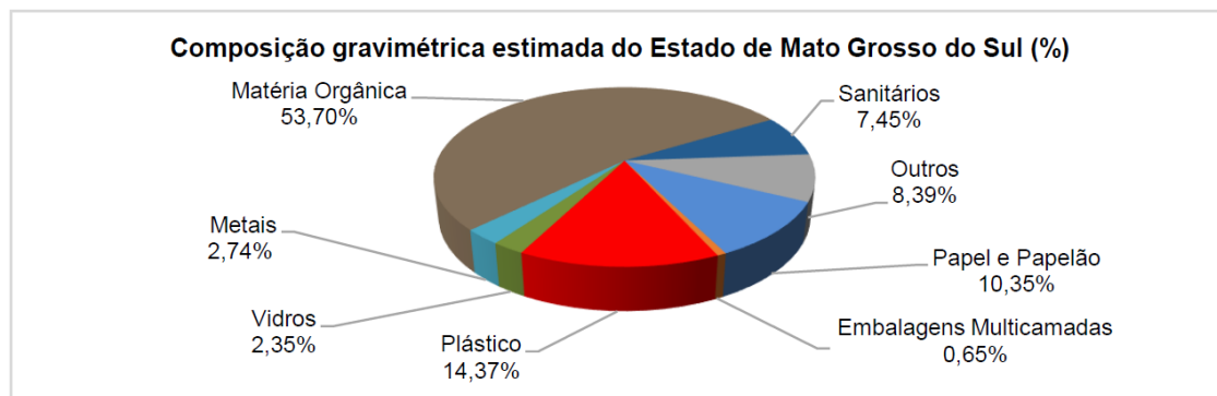
Figura 7: Composição gravimétrica estimada dos resíduos sólidos gerados no Estado de Mato Grosso do Sul. Fonte: (PERS-MS, 2020).
