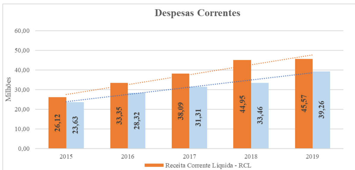
Gráfico 6: Comparação da RCL e das Despesas Correntes municipais de Paraíso das Águas.
