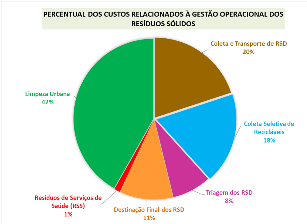
Gráfico 2: Percentual dos custos de cada serviço relacionados à gestão dos RS em Paraíso das Águas - MS.
