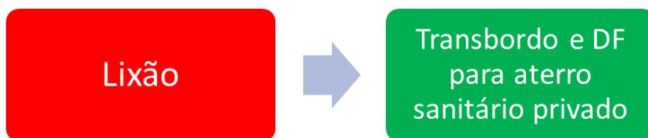
Figura 12: Situação da Destinação Final dos RSD em 2016 versus atual (2019).
