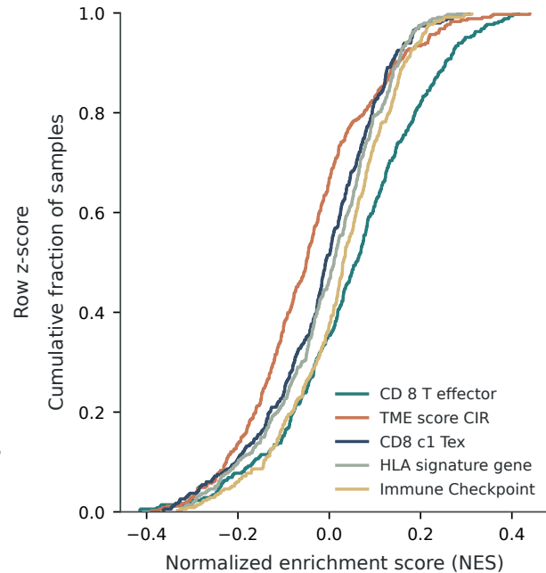
NES distributions · all 348 samples
