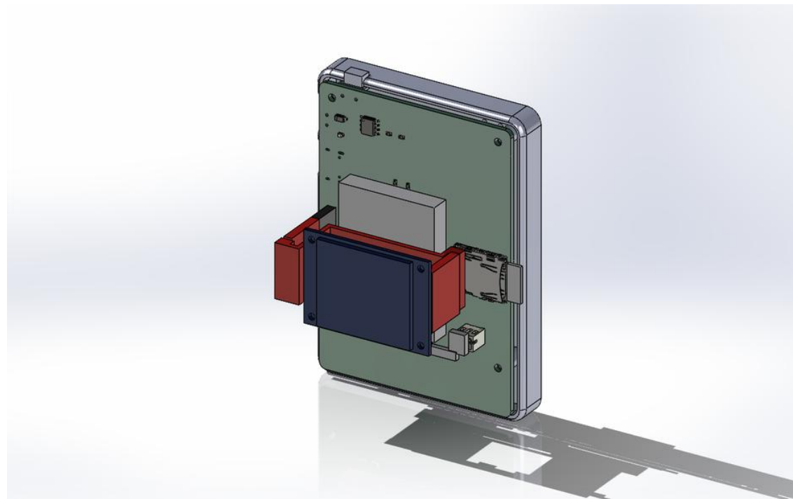
背面那片殼拿掉：紅色是接螢幕的杜邦線，螢幕鎖在殼上、蓋在電池上面
