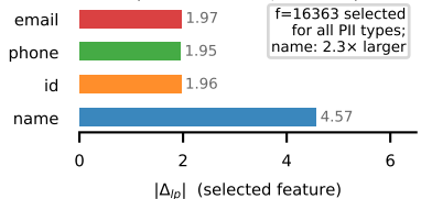
(d) Failure mode B: Llama L8 (same feature, all 4 PII)
