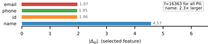
(d) Failure mode B: Llama L8 (all 4 PII types \rightarrow same feature)
