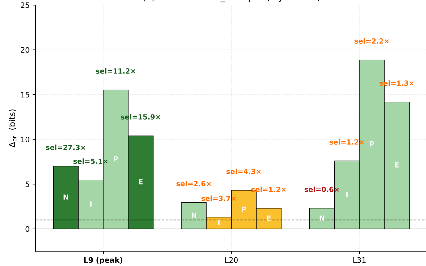
(d) Llama-Med42 — \Delta_{br} per (layer \times PII)
