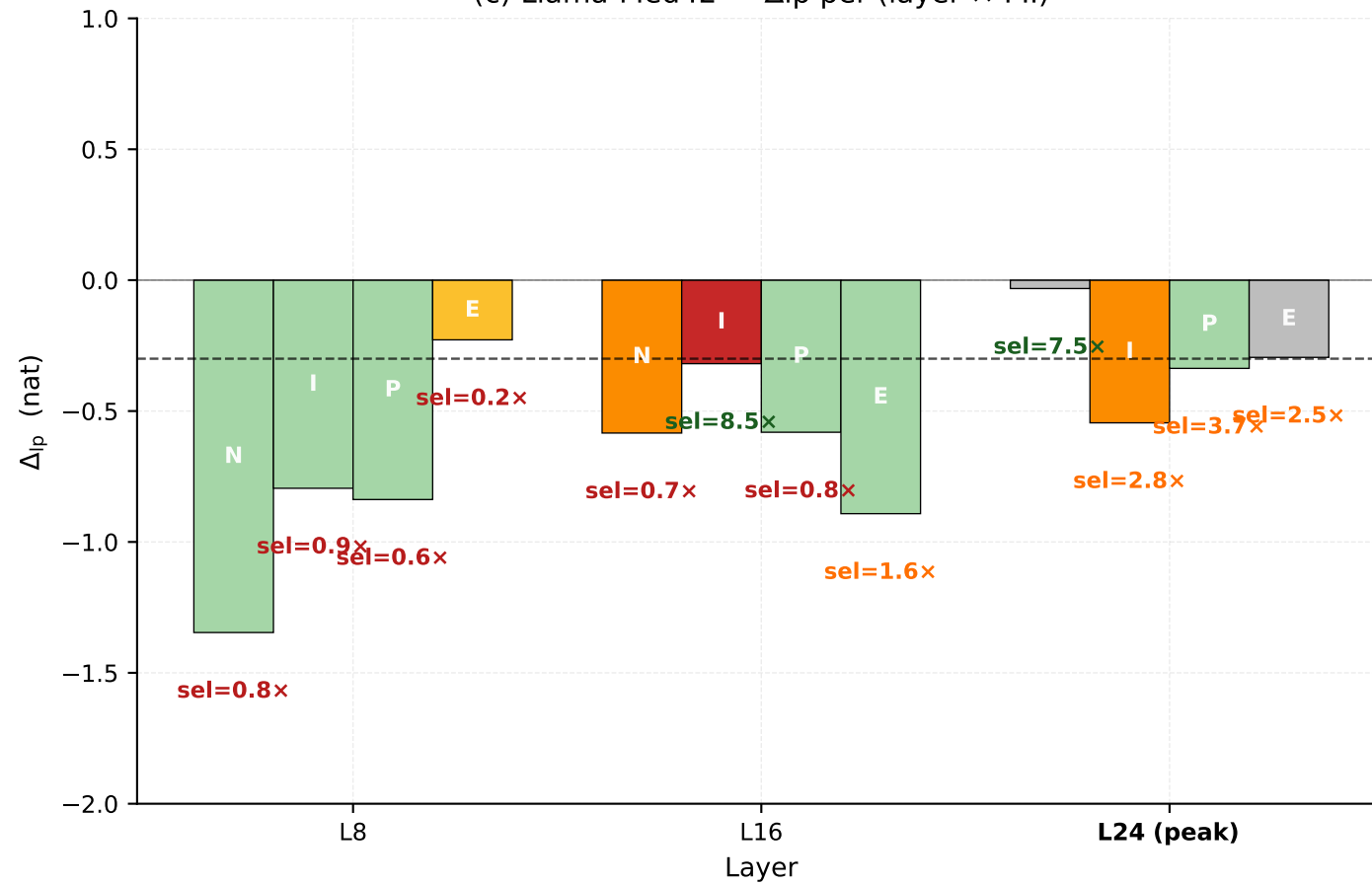
(c) Llama-Med42 — \Delta p per (layer \times PII)
