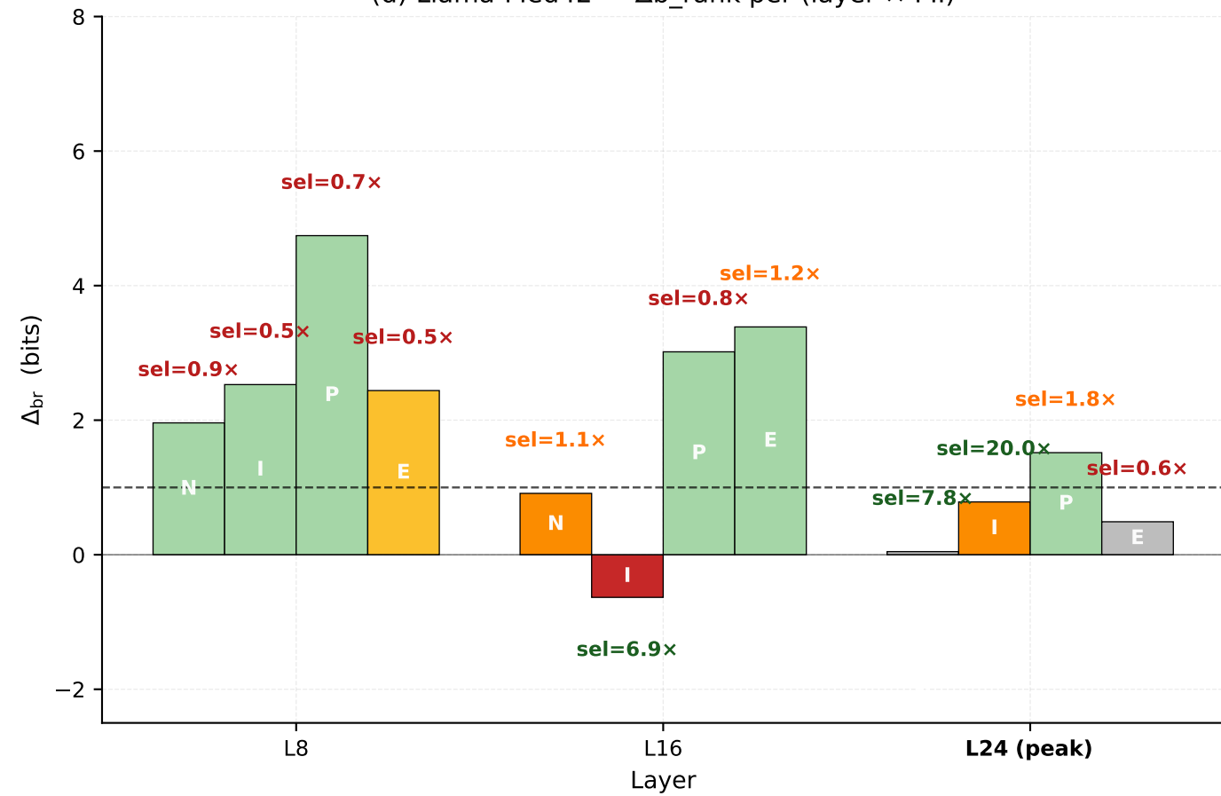
(d) Llama-Med42 — \Delta_{br} per (layer \times PII)
