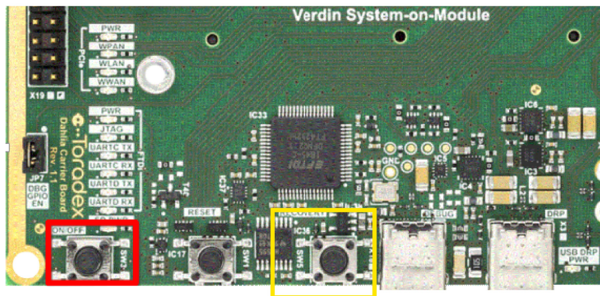
Fig 6. Ubicación botón RECOVERY.
