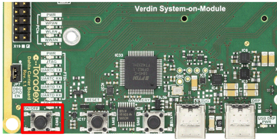
Fig 4. Ubicación botón ON/OFF.
