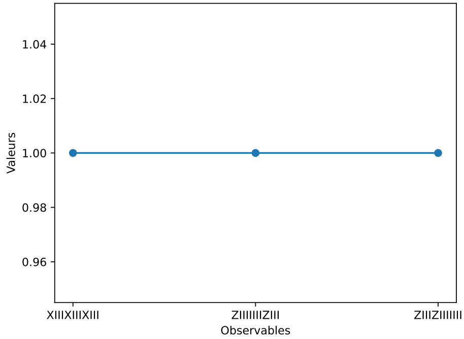
FIGURE 1 – Valeurs moyennes obtenues selon l'état GHZ simulé des stabilisateurs.
