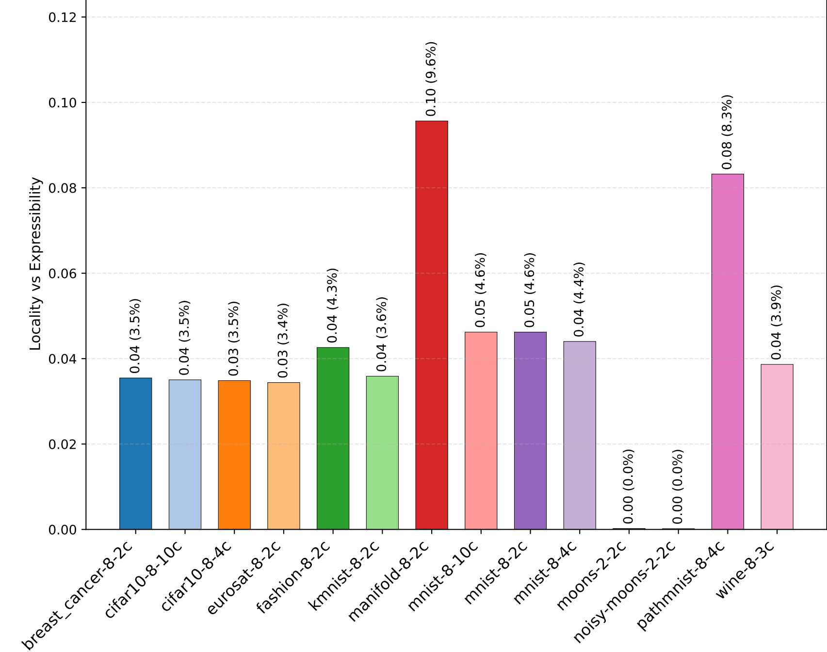
EGAS
