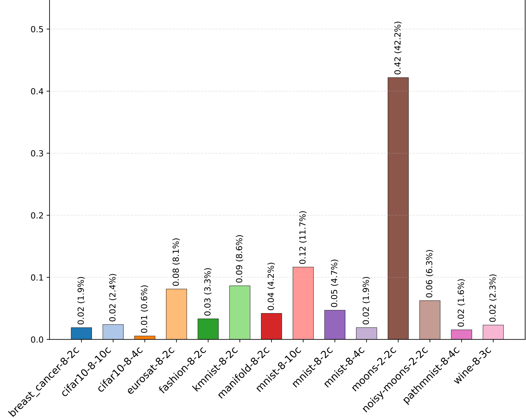
NQE
