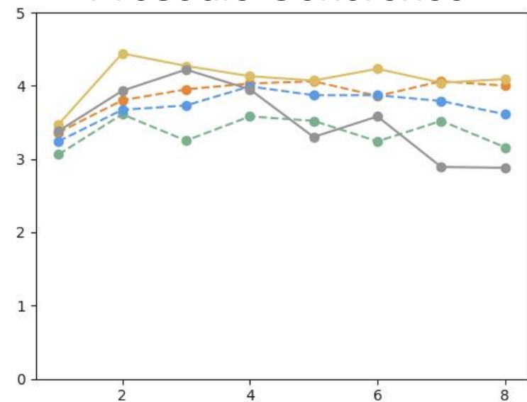
Prosodic Coherence
