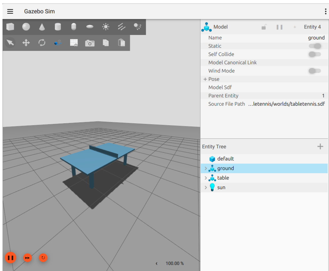
Abbildung 26.5: Die eingebundene Tischtennisplatte in Gazebo: korrekt in Metern skaliert (Spielfläche bei z = 0,76 m) und über Roll +90^\circ aufrecht gestellt. Sie bildet die Referenzgeometrie und die spätere Zielebene.
