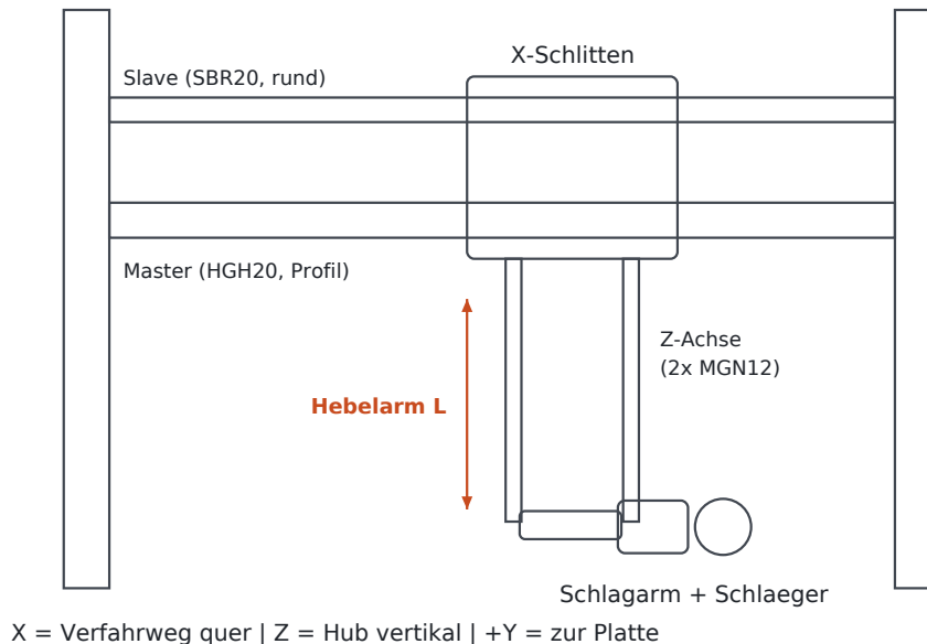
Abbildung 26.7: Frontblick auf das Portalkonzept: Der X-Schlitten greift die beiden vertikal gestapelten X-Schienen (Slave oben, Master unten); zwischen ihnen hängt die Z-Achse mit dem nach vorn ausladenden Schlagarm (Hebelarm L ).
