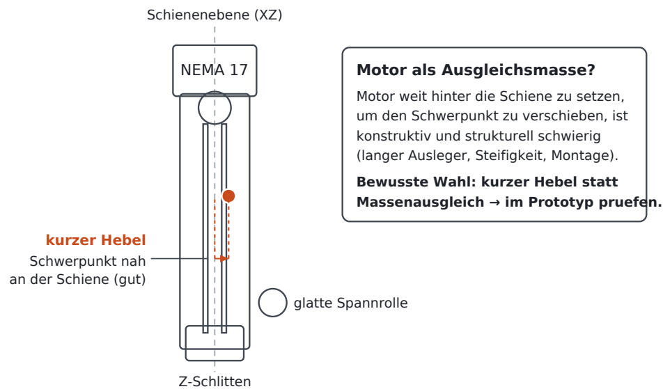
Abbildung 26.14: Bewertung der aktuellen Anbindung: Der NEMA 17 sitzt in der XZ-Schienenenebene mit kurzem Hebel; der Riemen läuft in der Ebene zum Z-Schlitten, eine glatte Spannrolle spannt. Der Motor als Ausgleichsmasse weit hinter der Schiene wäre konstruktiv schwierig – bewusst wurde der kurze Hebel gewählt und der Feinabgleich dem Prototyp überlassen.
