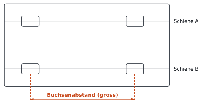
Abbildung 26.9: Draufsicht auf die Lageranordnung: zwei Wagen je Schiene, entlang X maximal gespreizt. Der große Buchsenabstand nimmt Nick- und Giermoment auf.
