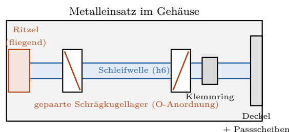
Abbildung 26.17: Querschnitt der Ritzelwelle (schematisch): Zwei gepaarte Schrägkugellager in O-Anordnung geben dem fliegenden Ritzel eine breite, momentensteife Stützbasis. Der Lagersitz liegt in einem Metalleinsatz (nicht im nackten Druckplastik), der Vorspannpfad läuft vollständig durch Metall; Deckel und Passscheiben stellen Position und Zahnflankenspiel ein.
