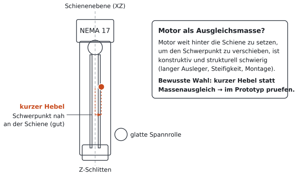
Abbildung 26.14: Bewertung der aktuellen Anbindung: Der NEMA 17 sitzt in der XZ-Schienebene mit kurzem Hebel; der Riemen läuft in der Ebene zum Z-Schlitten, eine glatte Spannrolle spannt. Der Motor als Ausgleichsmasse weit hinter der Schiene wäre konstruktiv schwierig – bewusst wurde der kurze Hebel gewählt und der Feinabgleich dem Prototyp überlassen.
