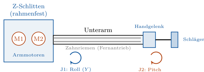
Abbildung 26.15: Fernantrieb-Schema des 2-Gelenk-Handgelenks: Beide Motoren bleiben rahmenfest auf dem Z-Schlitten, die Kraft läuft über Zahnriemen den Unterarm entlang. J1 rollt den Unterarm um seine Längsachse (Vorhand/Rückhand), J2 führt den Pitch-Schlag; distal wird nur noch geringe Masse beschleunigt.
