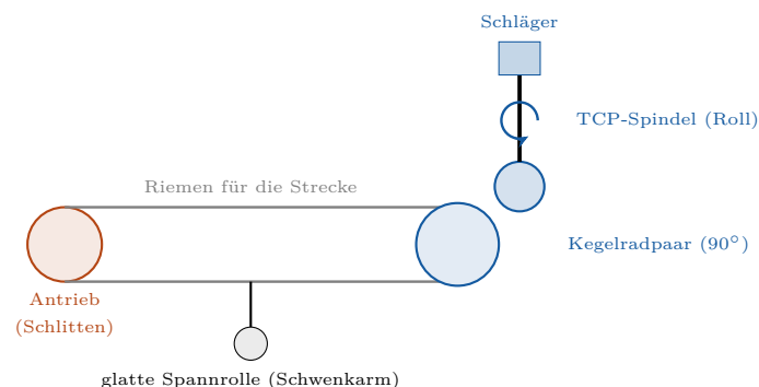
Abbildung 26.16: Riemenführung und 90°-Umlenkung: Der Riemen überbrückt die Strecke vom Schlitten zur Kegelradwelle, das Kegel-/Miterradpaar lenkt die Drehung um 90° auf die TCP-Spindel um („Kegelrad für die Ecke, Riemen für die Strecke“). Die glatte Spannrolle sitzt frei auf einem Schwenkarm, nicht kollinear zu einer Achse.
