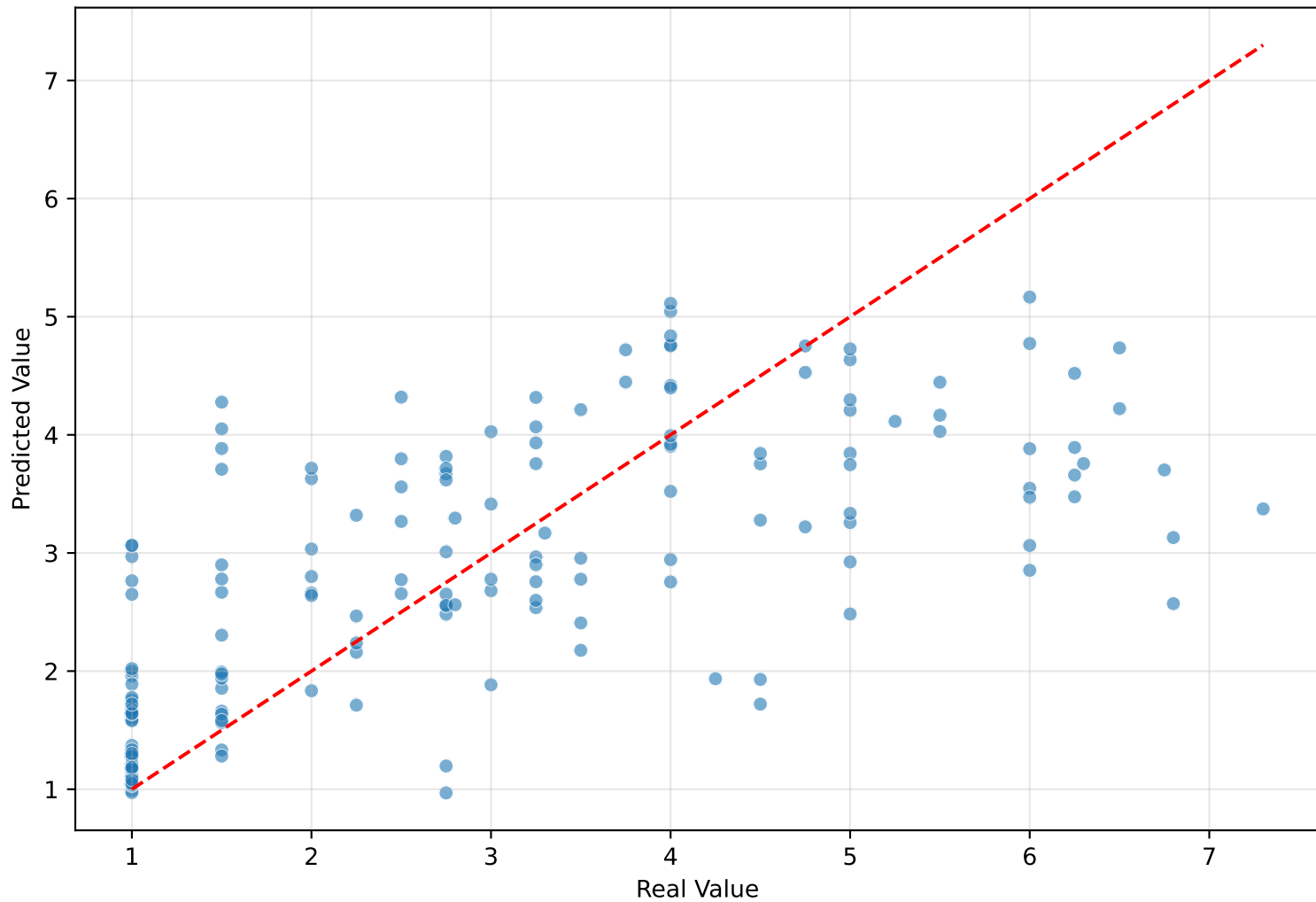
CNN MSE: 1.7167 - R 2 : 0.4540
