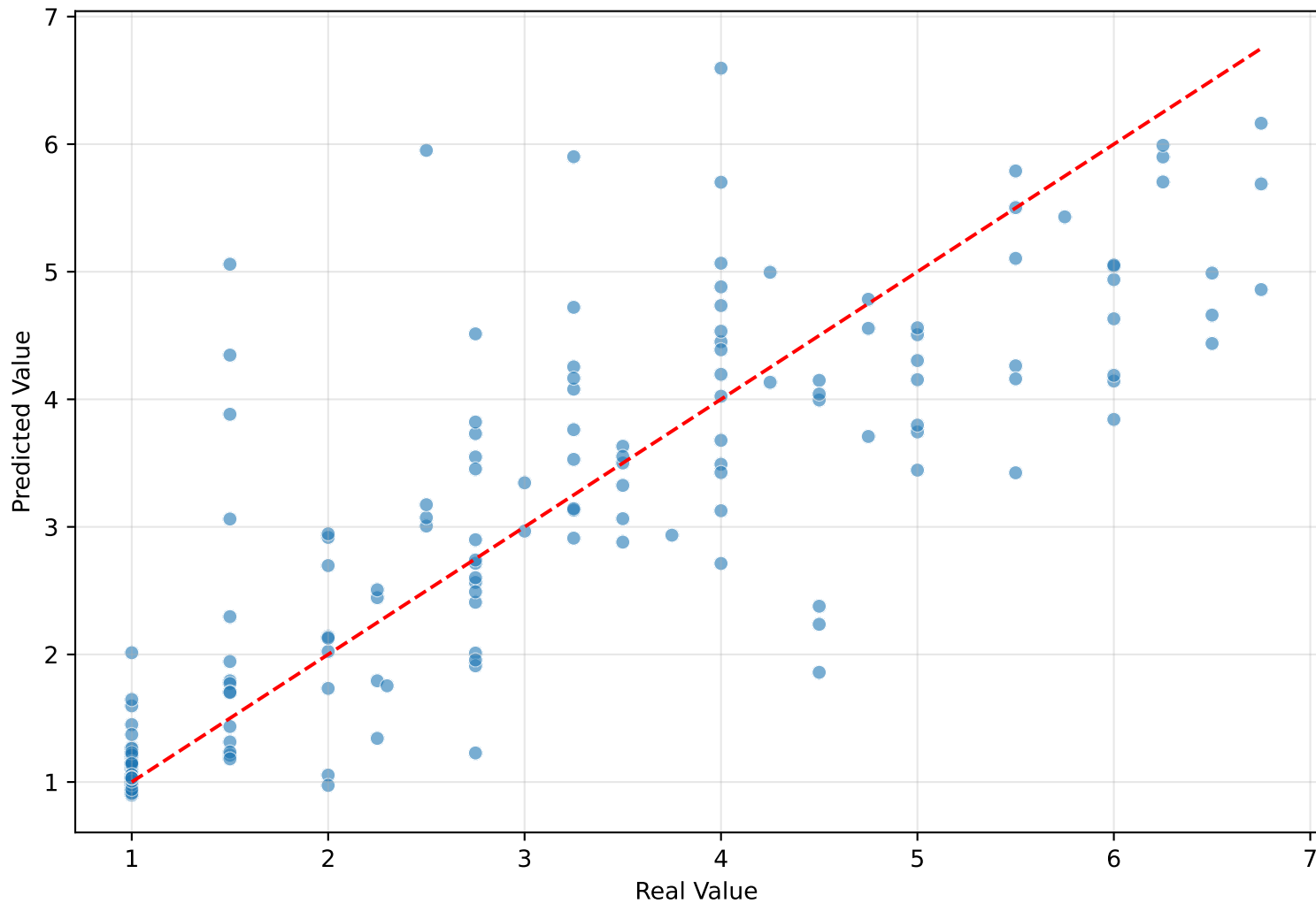
CatBoost MSE: 0.9373 - R 2 : 0.6933
