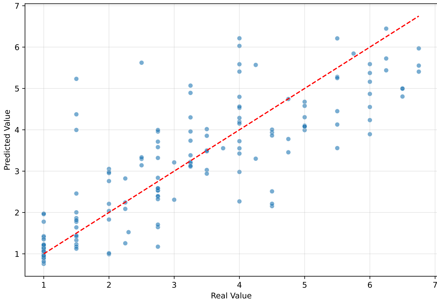
NGBoost MSE: 0.8873 - R 2 : 0.7097
