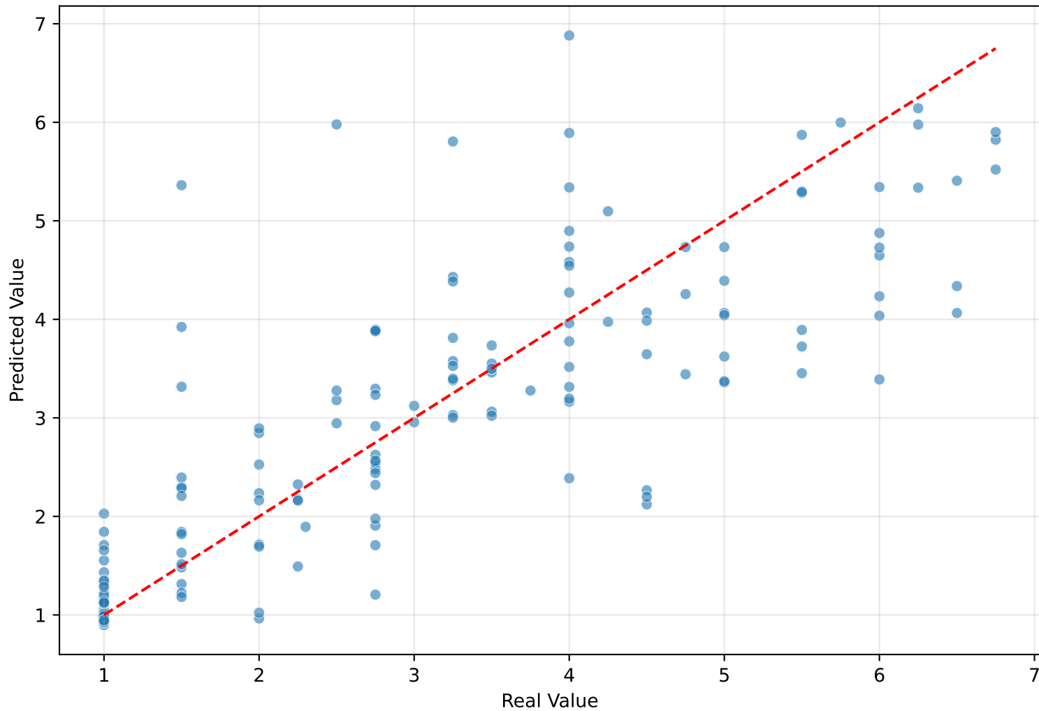
XGBoost MSE: 0.9768 - R 2 : 0.6804
