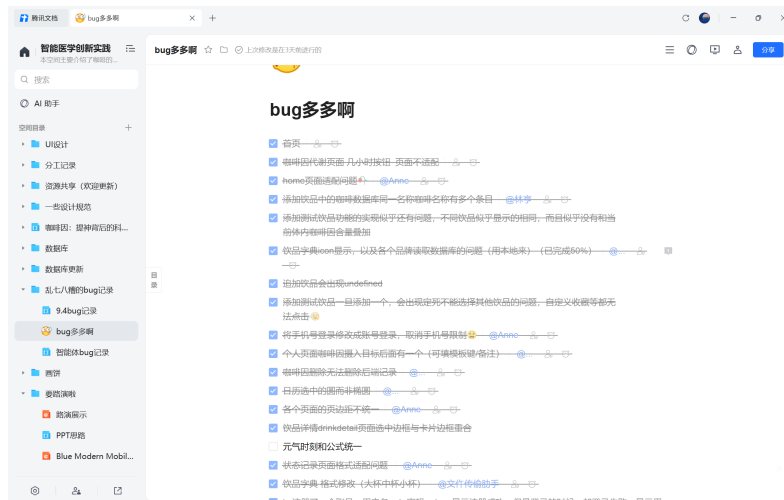
图 10: bug 修复 1
