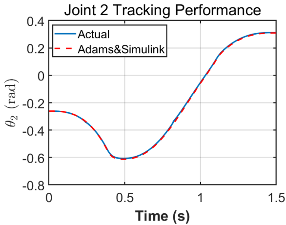
(b)关节 2 (b)Joint 2
