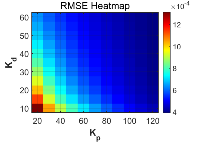
图 8 控制增益对跟踪精度的影响
