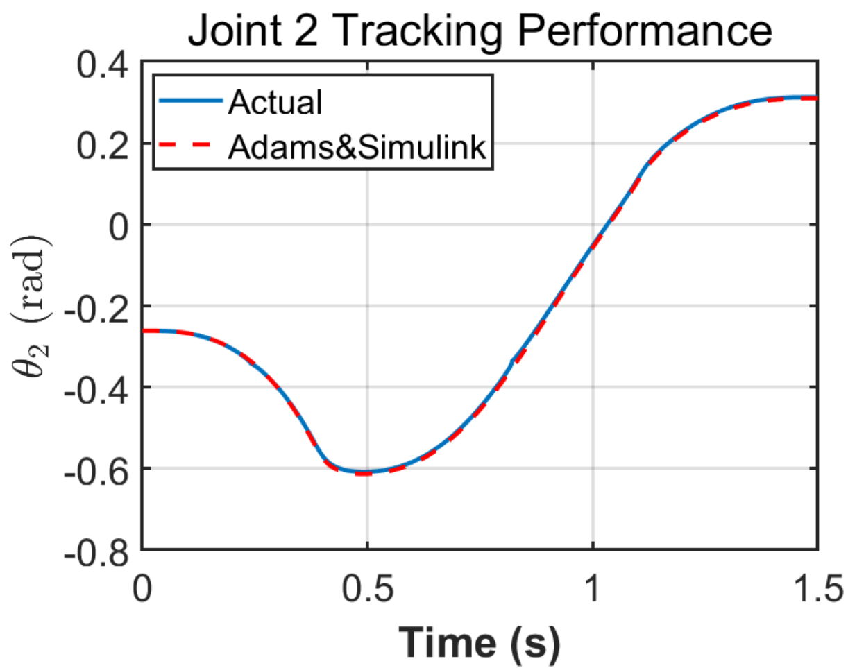
图 6 (b)
