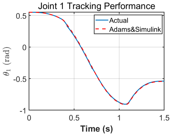
(a)关节 1 (a)Joint 1
