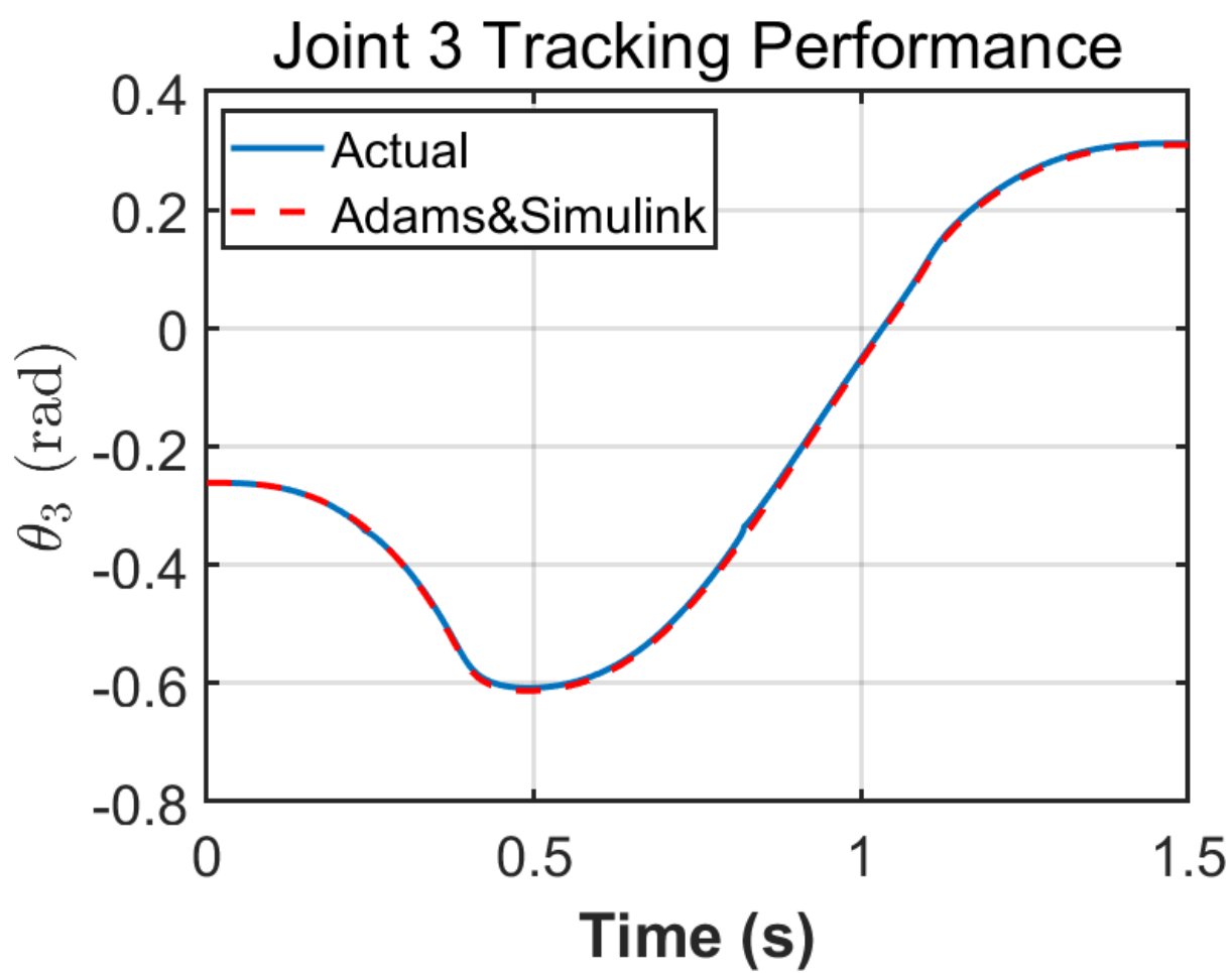
图 6 (c)
