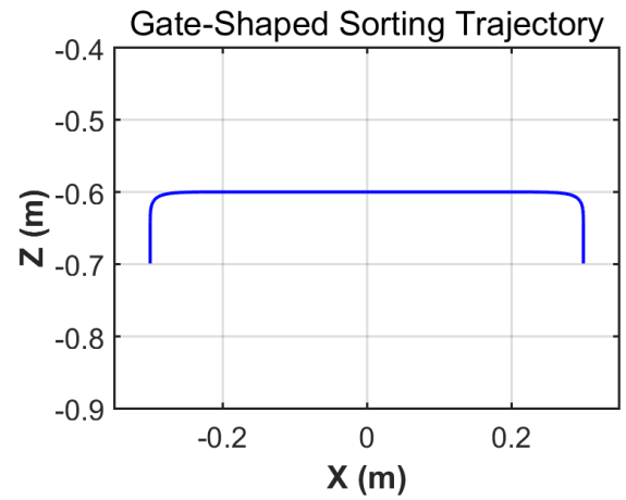
图 4 基于 PH 曲线的分拣轨迹
