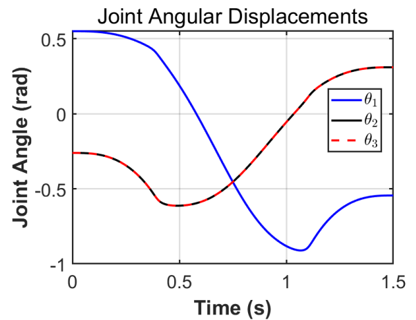
(a) 关节位移轨迹
