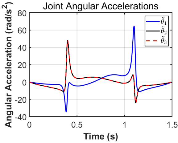
(c) 关节加速度轨迹
