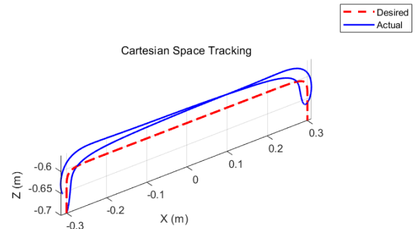
(a) 纯 PD 控制
