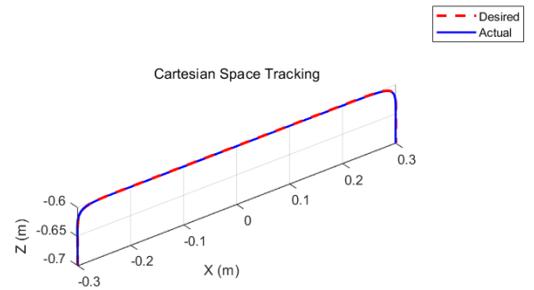
(b) 前馈动力学补偿的 PD 控制
