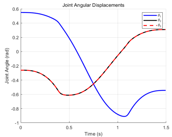
(a) 关节位移轨迹
