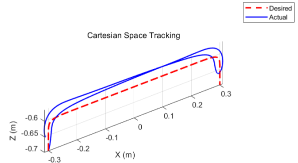
(a) 纯 PD 控制 (a) Only PD control
