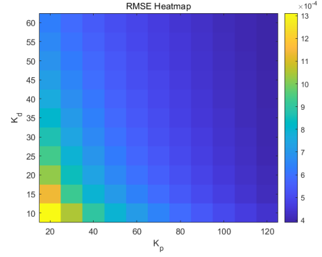
图 8 控制增益对跟踪精度的影响
