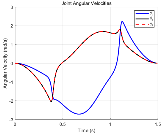
(b) 关节速度轨迹
