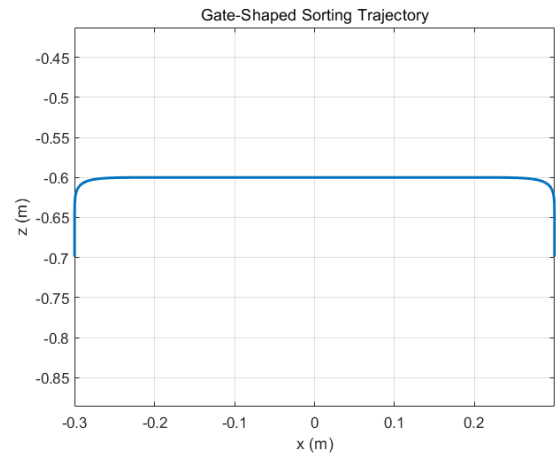
图 4 基于 PH 曲线的分拣轨迹
