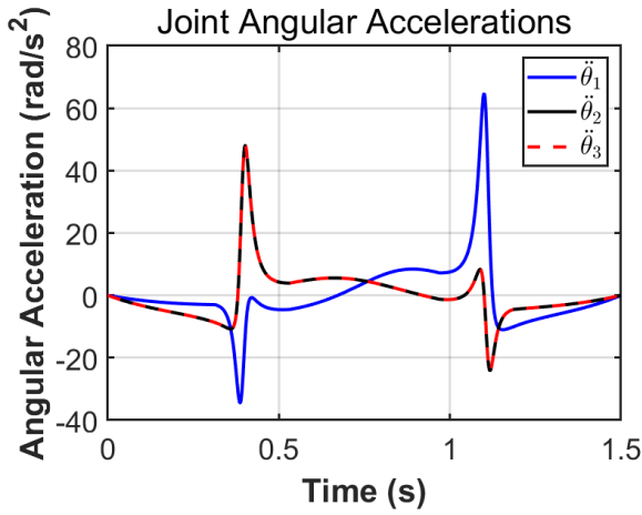
(c) 关节加速度轨迹
