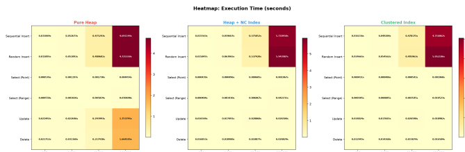
Fig. 3. 인덱스 구조와 연산 간의 성능 차이 (히트맵)
