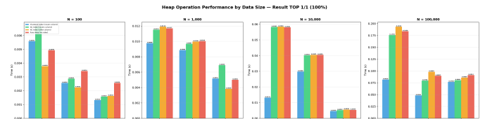
Fig. 4. 힙 연산(ORDER BY, GROUP BY, JOIN) 종류에 따른 소요 시간 비교
