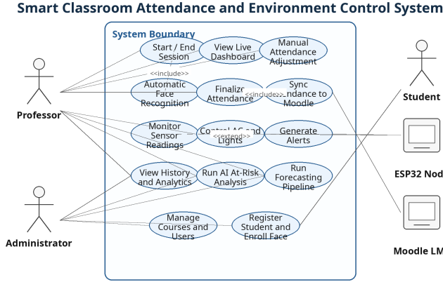
Fig. 1. UML use case diagram.
