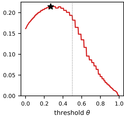
SVD Py
