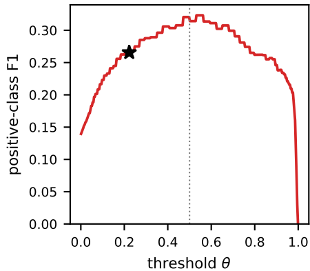
SVD Java
