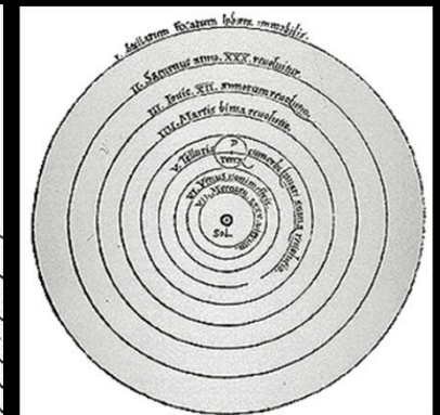
Heliocentrisme
