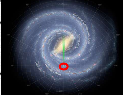
Jordens position i galaksen
