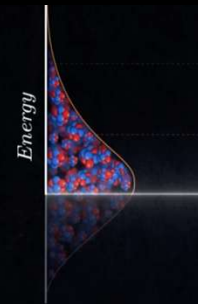
Energitilstande af atomerne
