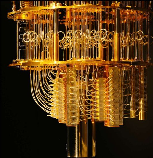
Kvantecomputer
