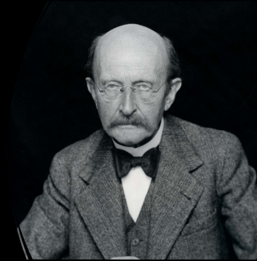
Max Planck (1858–1947)
