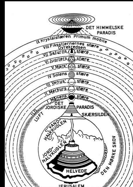
Geocentrisme
