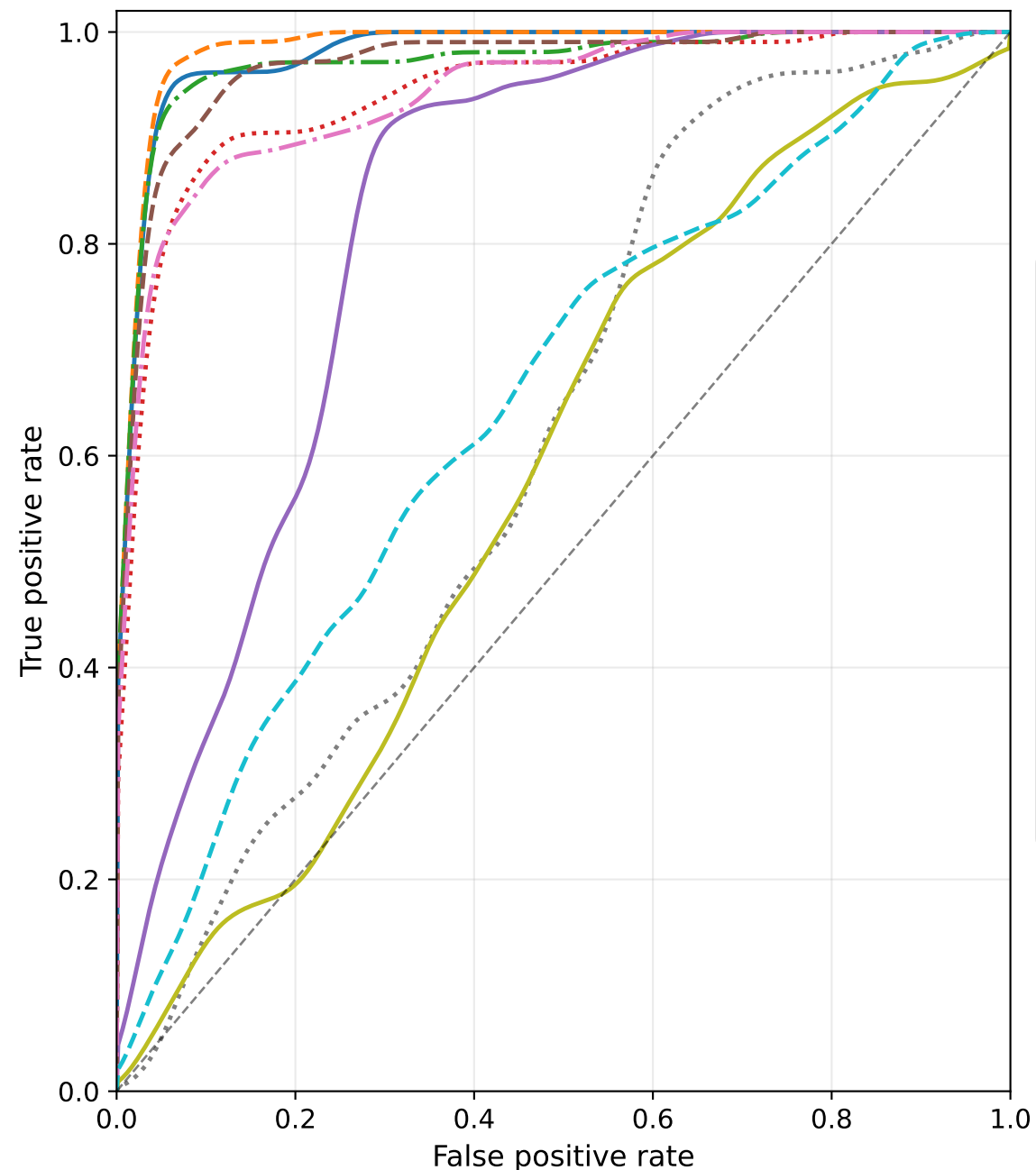
(b) ROC
