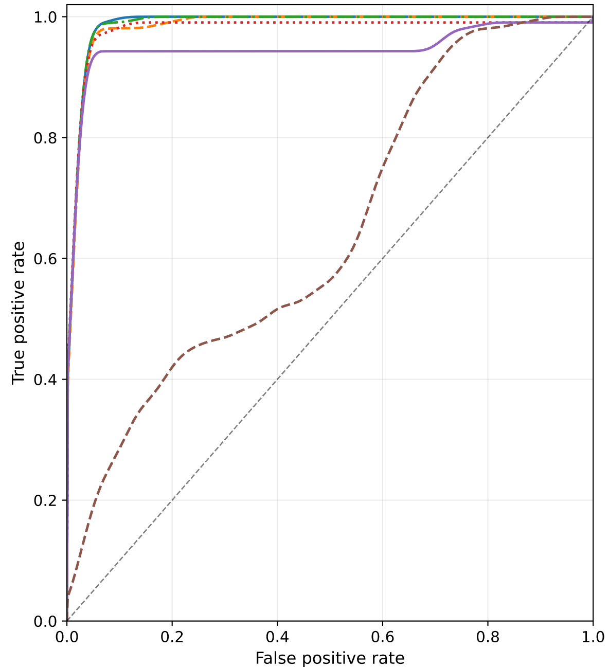
(b) ROC
