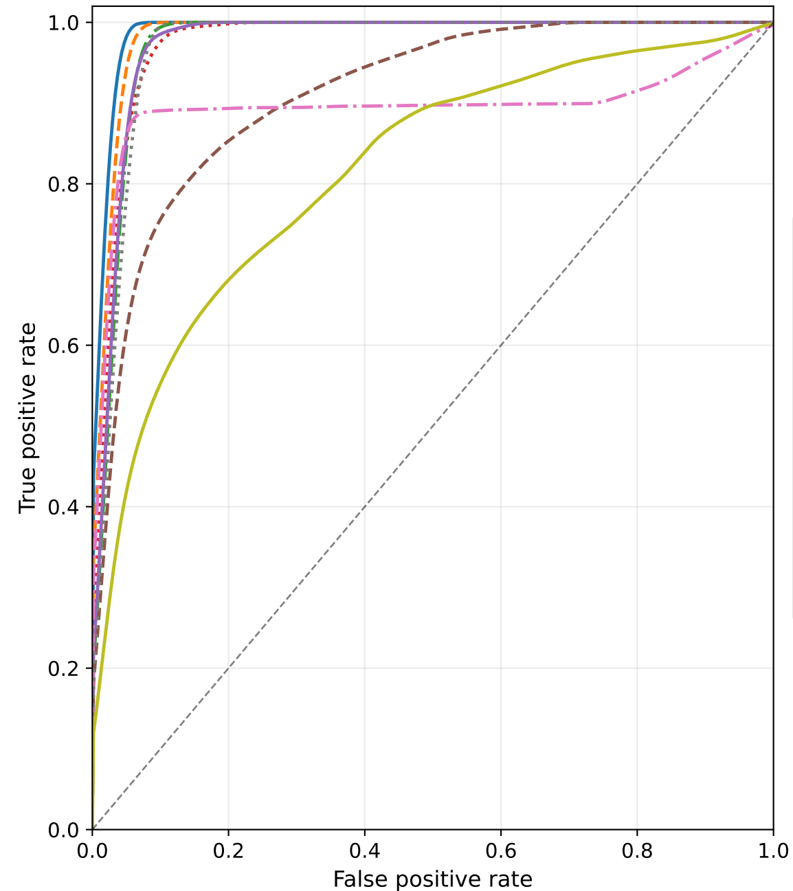
(b) ROC
