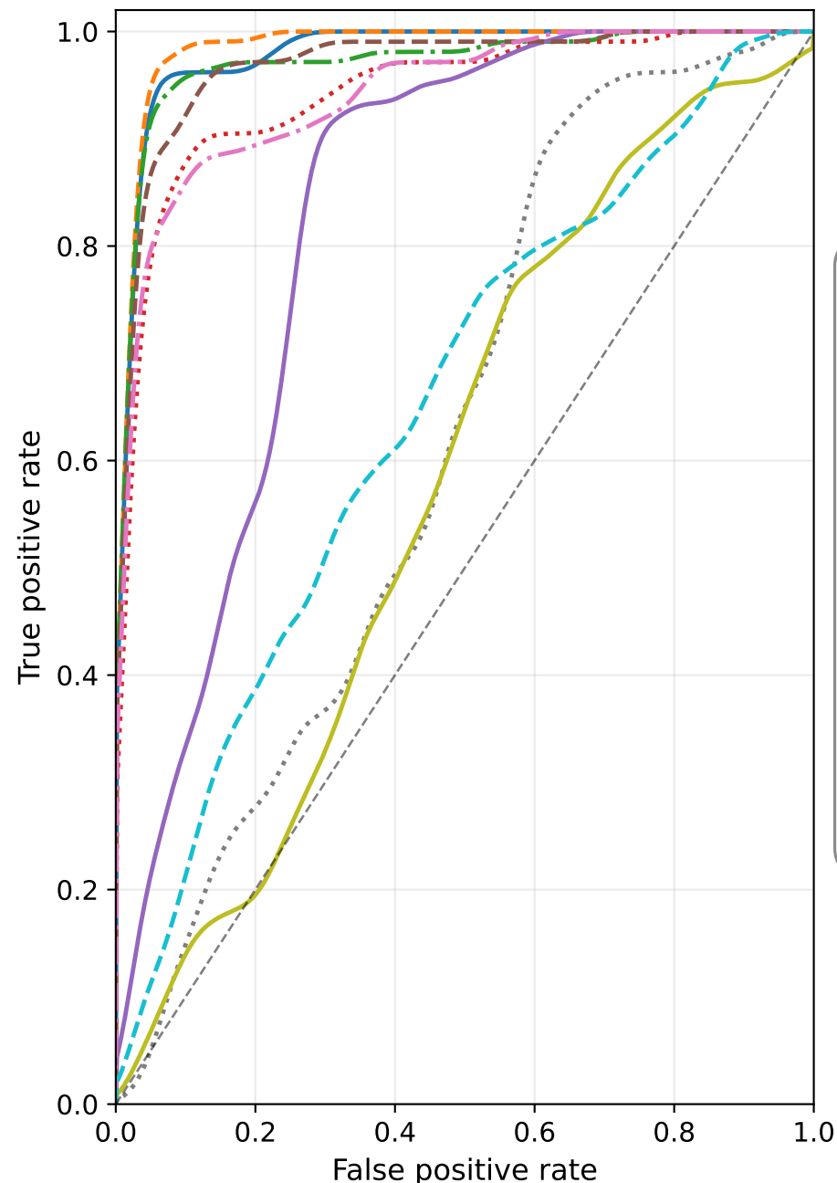
(b) ROC
