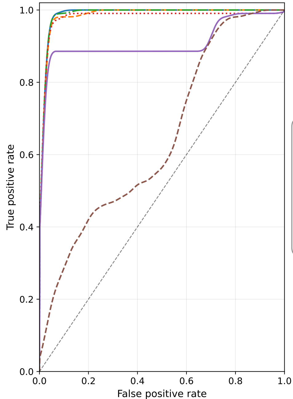
(b) ROC
