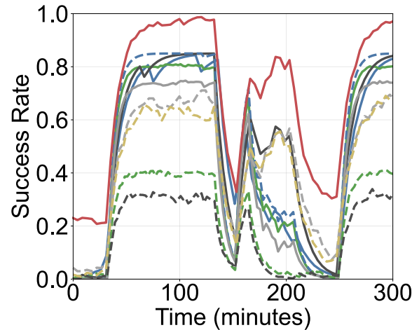
(d) Humanoid robot Baselines / VLASelect avg. acc: 0.4275 / 0.7245 (29.70%↑)
