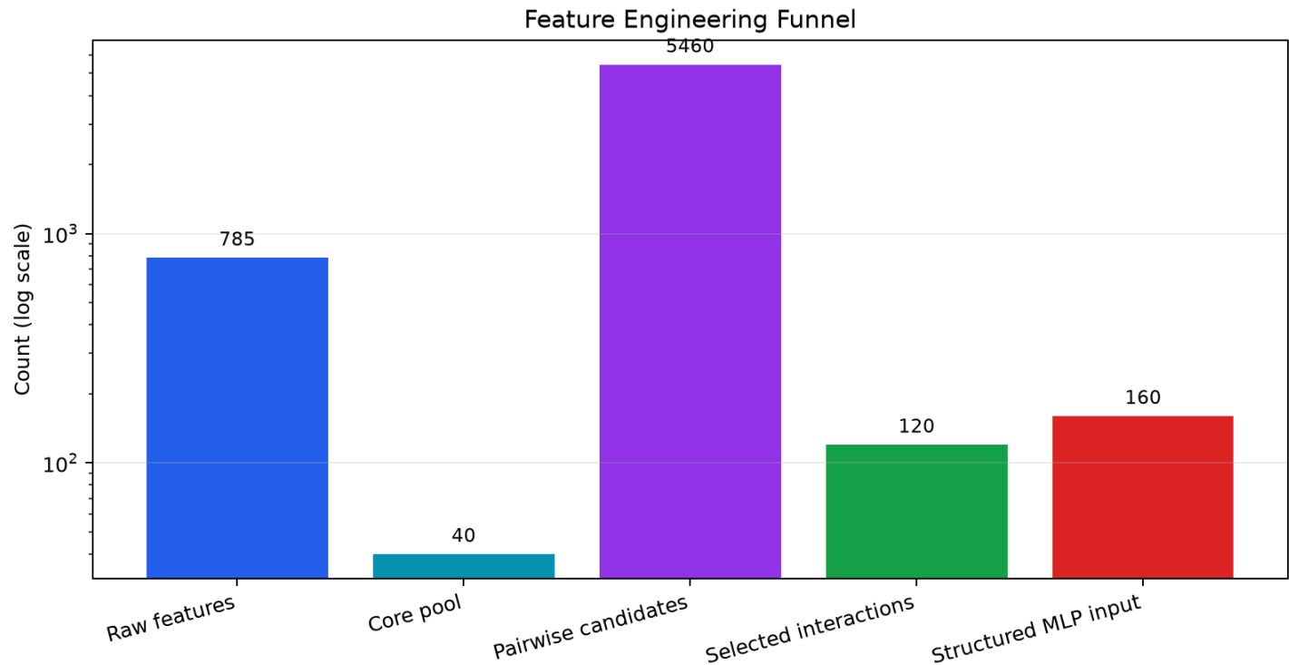
图 1 特征工程漏斗
