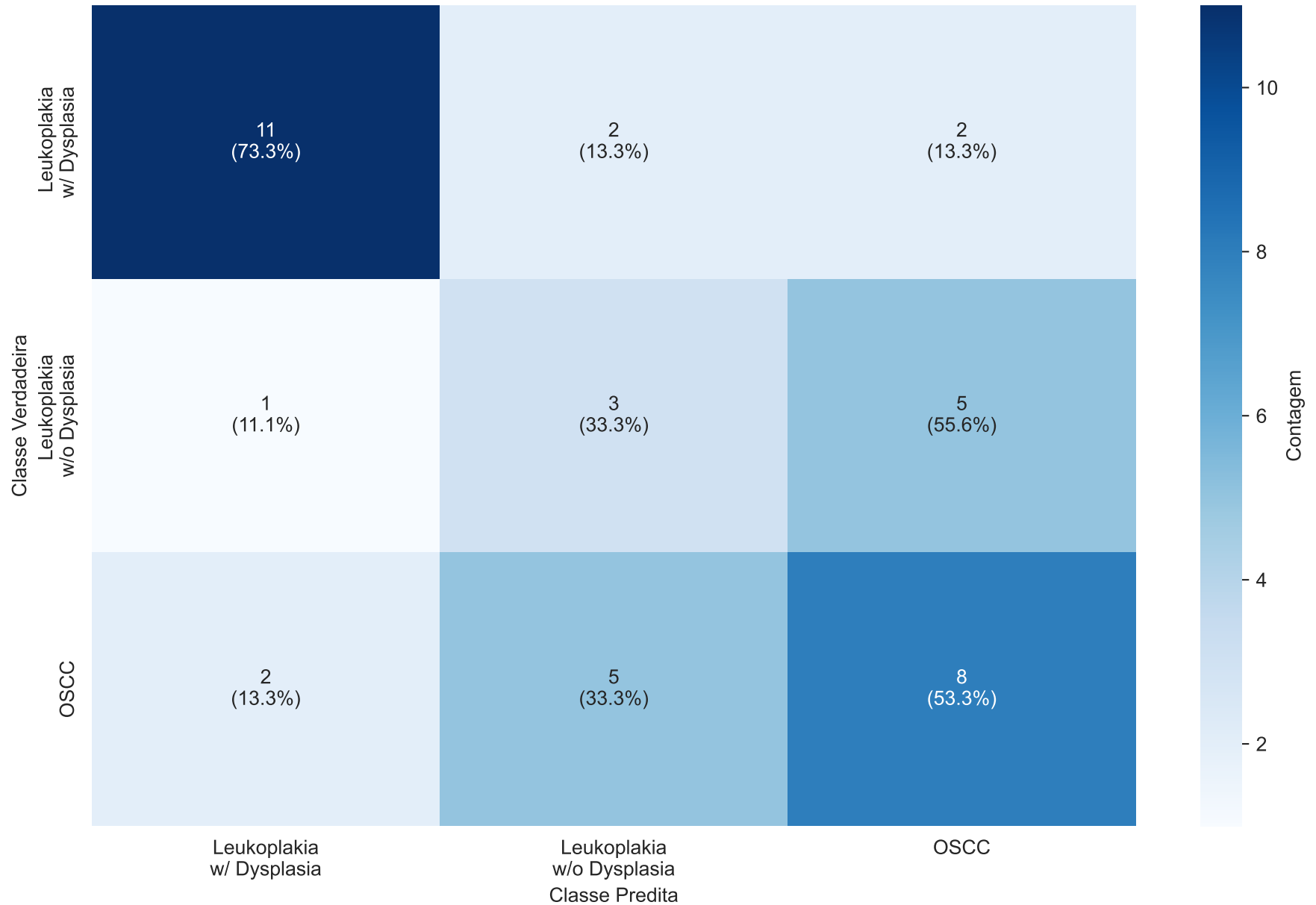
Matriz de Confusão — NDB-UFES EfficientnetV2_B0 | feature_extraction | Sem Aug | Seed: 42
