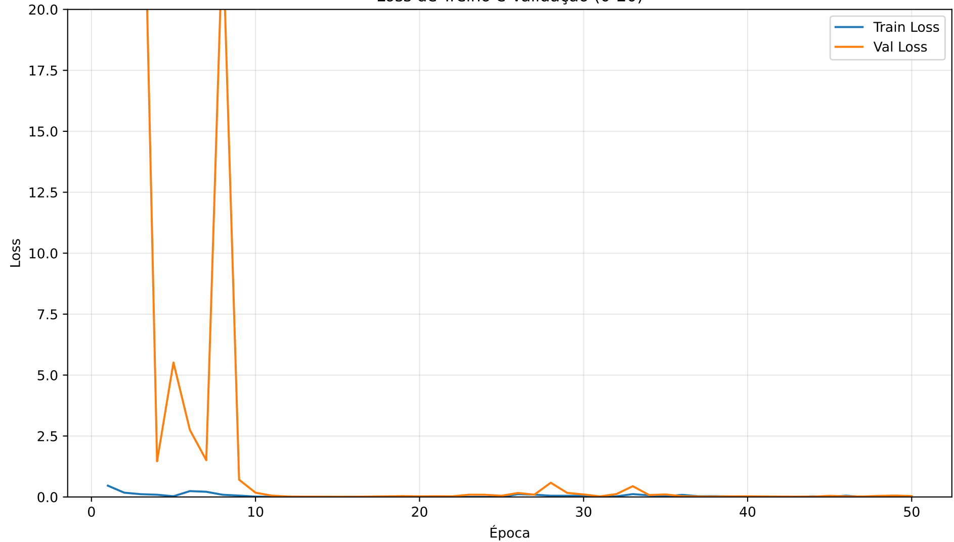
Loss de Treino e Validação (0-20)
