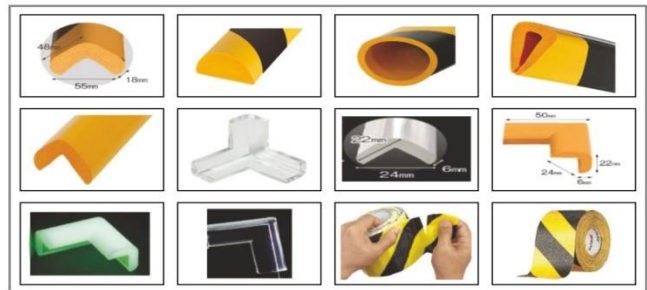
SIREN
