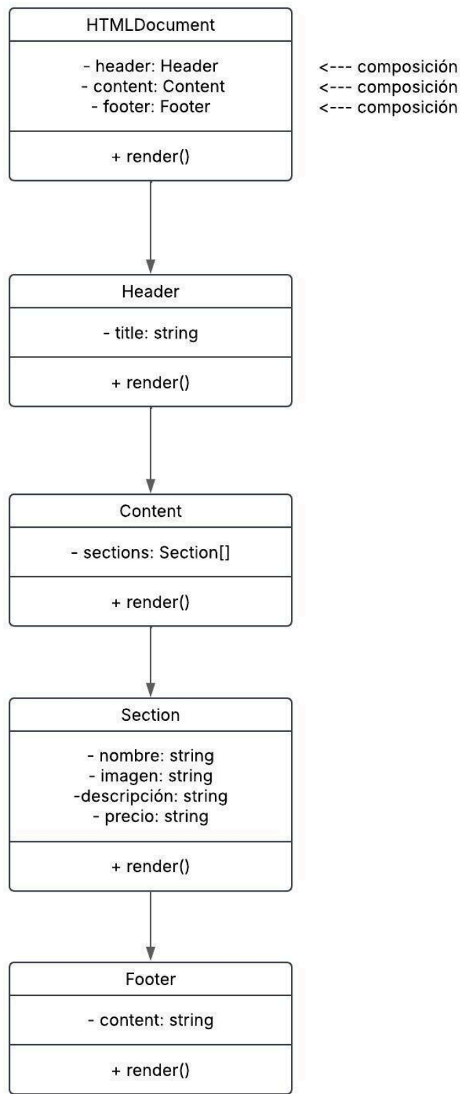
Diagrama UML
